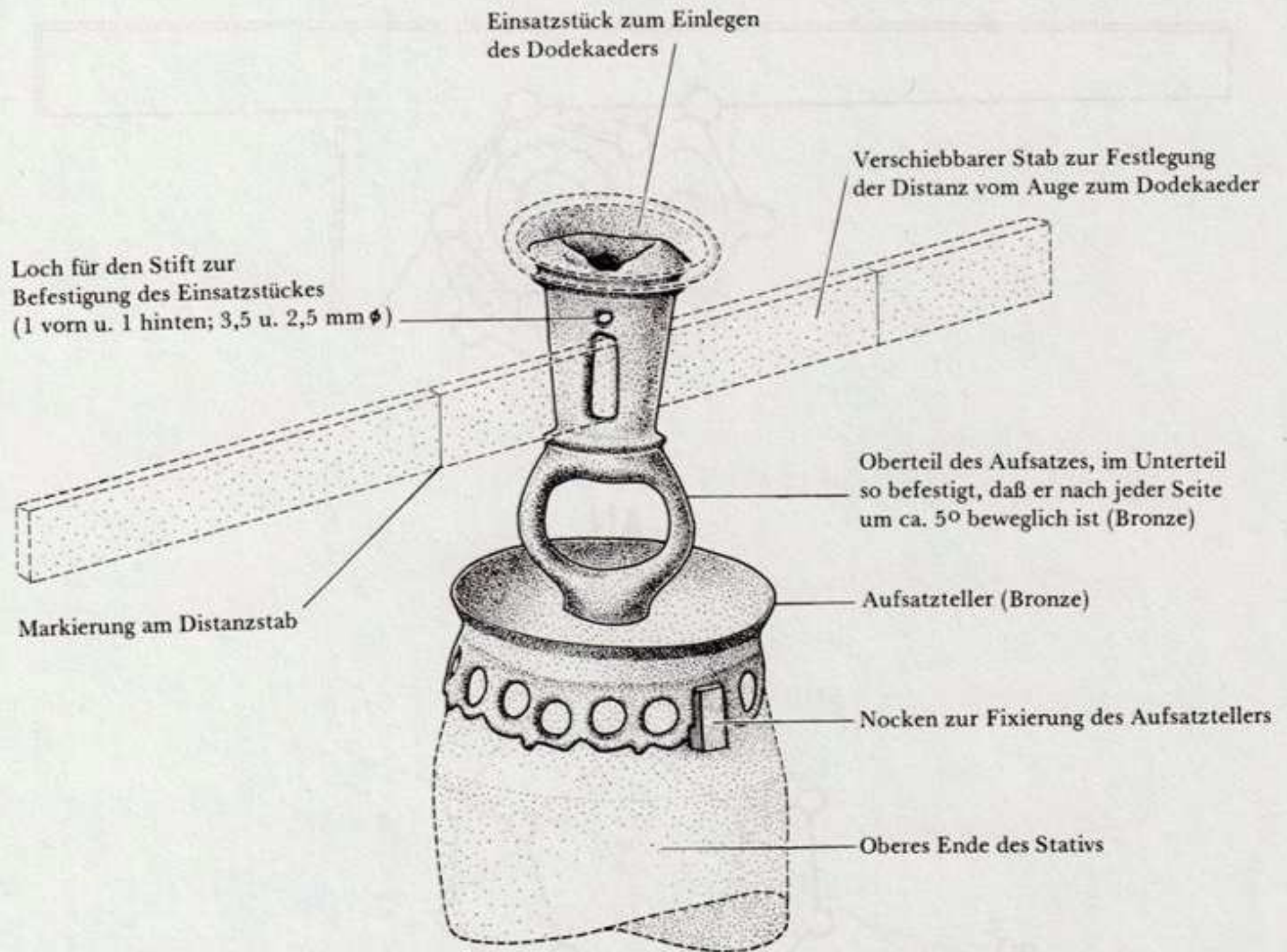
Abb. 3 Rekonstruktion des Zusatzgerätes für das Pentagon-Dodekaeder als Entfernungsmesser.
